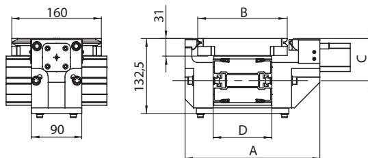
Index orizzontale per pallet senza tomini doneo per utilizzo con stop 85650901/2/3/4 Horizontal indexing unit for pallet without guide base arranged for stop unit 85650901/2/3/4
